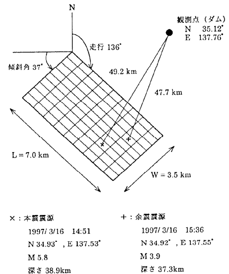
図-1 断層モデル及び観測点
