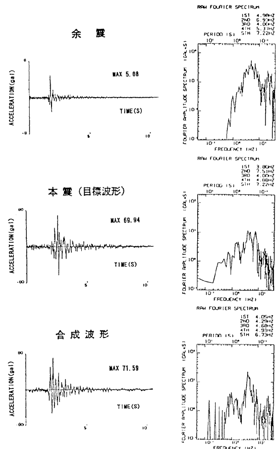
図-2 ダム右岸における余震, 本震, 合成波形 (時刻歴波形, 周波数特性: 上下成分)
