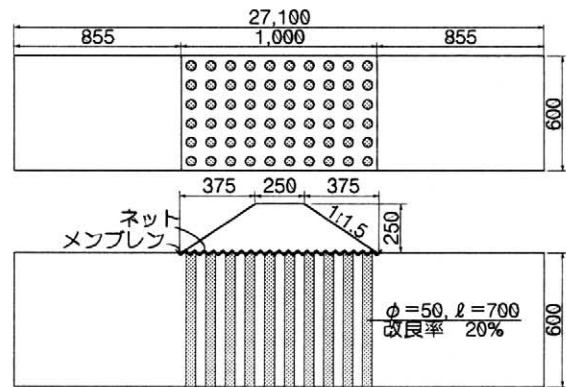
図-2 地盤改良の配置概要
