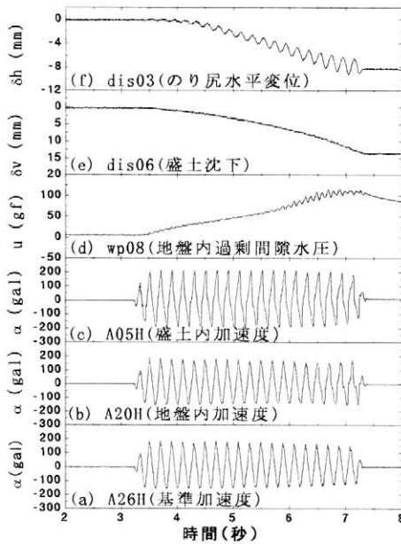
図4 無対策ケース
