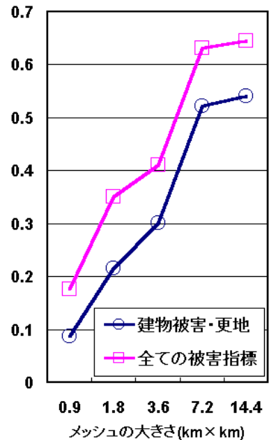
図 3: 四分位連関係数と、被災指標グループ、メッシュの大きさの関係
