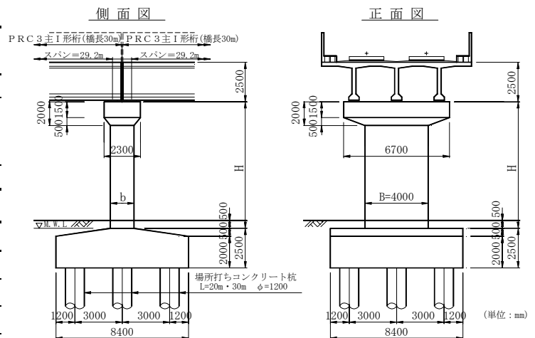
図-1 杭基礎RC橋脚の形状寸法
