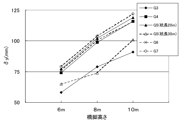
図-2 構造物全体系の降伏変位 \delta y
