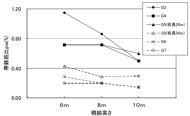
図-5 帯鉄筋比 p_w
