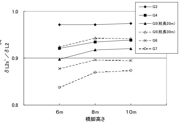
図-4 \delta L2 における \delta L2s' の占める割合
