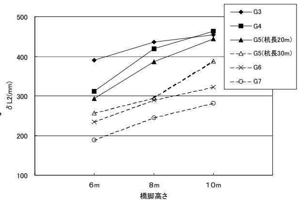
図-3 L2 地震動による構造物の応答値
