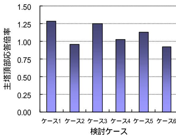
図-4 免震ケースによる塔頂変位比較
