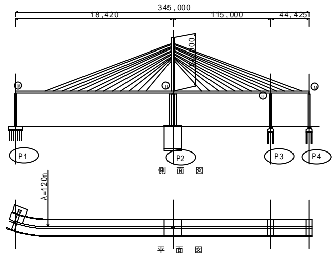
図-1 対象橋梁概略図
