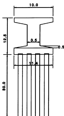
図-1 橋脚図
