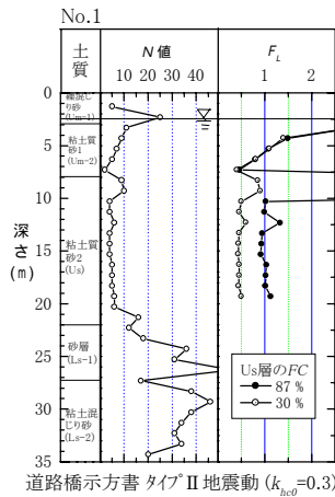
図-3 地盤柱状図
