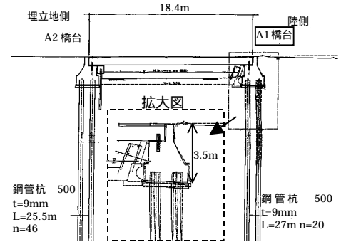
図-2 断面図
