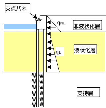
図-4 解析モデルの概念図
