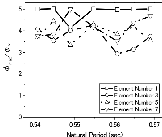
Fig.3 最大曲率と降伏曲率の比
