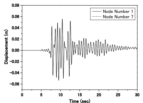
Fig.2 時刻歴応答(変位)
