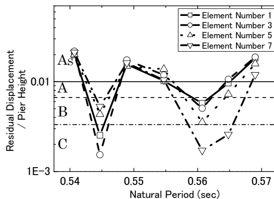
Fig.5 橋脚限界値
