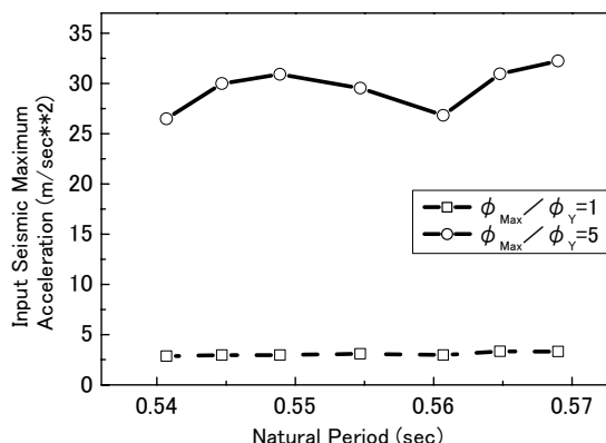
Fig.4 入力地震動の最大加速度
