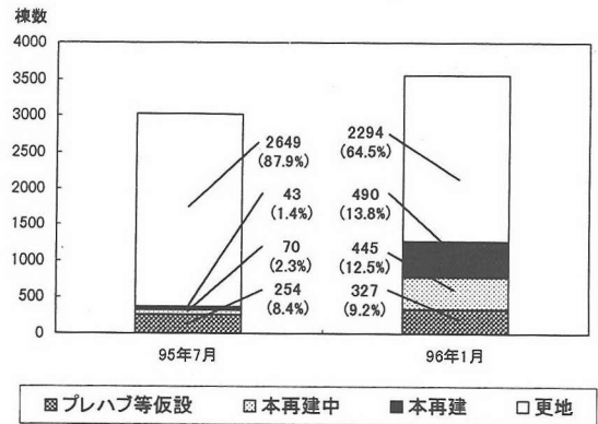
図-7 被災建物の再建棟数(対象地域全体)
