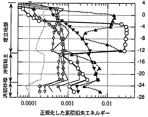
図-12 正規化累積損失エネルギーの深さ方向分布
