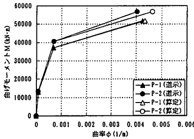
図-11 M~φ曲線(プレート境界型)
