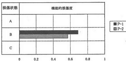
図-22 内陸直下型地震動における鋼板巻立て補強およびヒューズ支承を適用したP-1, 2の全体系機能的損傷度
