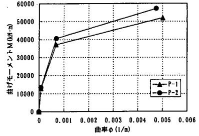
図-5 M~φ関係(内陸直下型)
