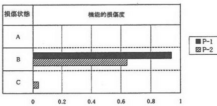
図-20 内陸直下型地震動における鋼板巻立て補強を施したP-1, 2の全体系機能的損傷度
