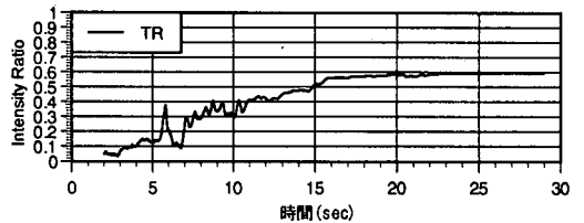
図-20 Arias Intensity 比 (尼崎高架橋)
