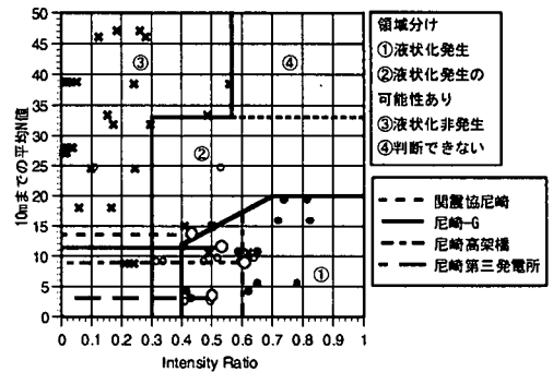
図-22 平均 N 値と Intensity 比の関係
