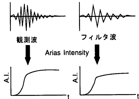
図-2 Arias Intensity の算定
