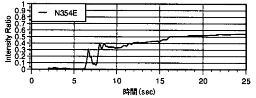
図-18 Arias Intensity 比 (尼崎-G)
