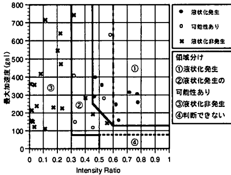
図-9 最大加速度値と Intensity 比の関係
