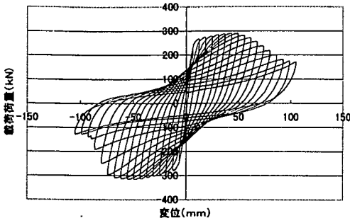
図-5 III-1の荷重変位曲線
