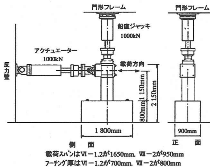
図-3 荷重装置概要
