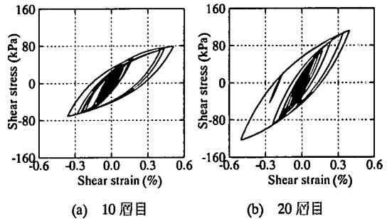
図-4 応力-ひずみ関係
