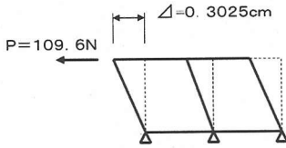
図-5 トンネルの荷重試験概要図
