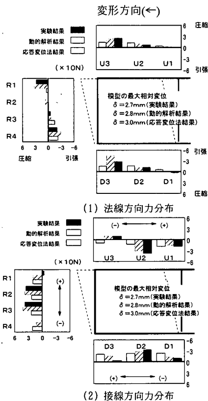
図-20 相互作用力分布(解析結果)
