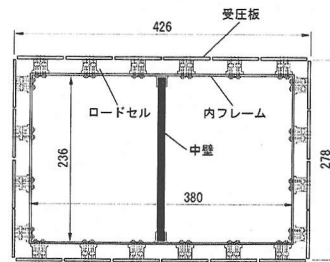
図-3 模型トンネル断面図（2径間）
