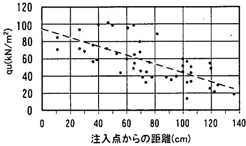
図-10 注入センターからの距離と q_u の関係
