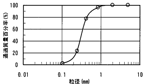
図-5 新潟砂の粒度分布
