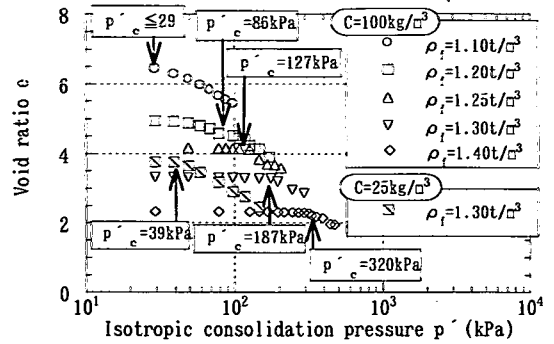
図-13 配合の異なる試料の初期状態での e \sim \log p' 曲線
