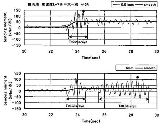
図-22 中央杭頭モーメント時刻歴(大一別)
