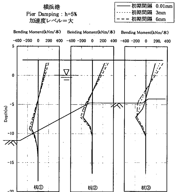
図-19 栈橋杭の曲げモーメント分布
