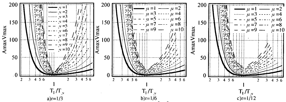
図-9 塑性率毎の最大値指標( A_{\max} V_{\max} : \text{m}^2 / \text{s}^2 )と規準化された周期の関係
