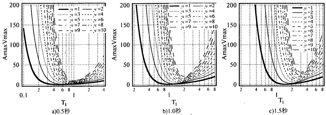
図-8 固有周期に応じた塑性率毎の最大値指標( A_{\max} V_{\max} : \text{m}^2 / \text{s}^3 )と入力波の周期( T_i : \text{sec} )の関係(剛性比 r = 1/6 )
