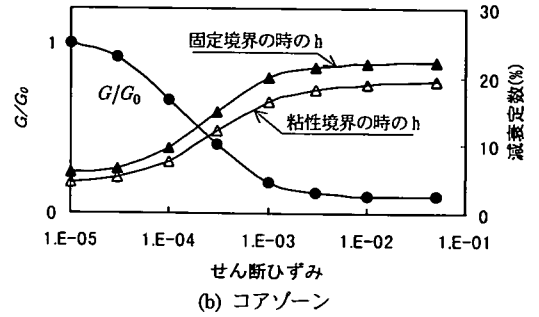
図-27 側方の境界条件に応じたV字谷モデルの等価せん断剛性比と減衰定数
