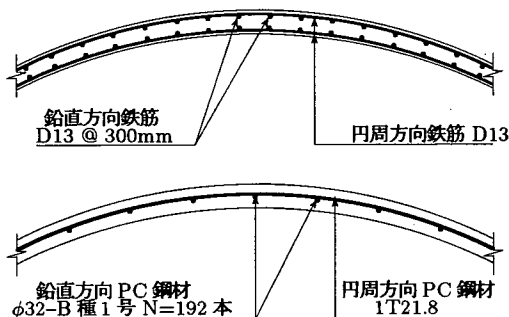
図-3 基準タンク側壁の配筋図 (鉛直方向)
