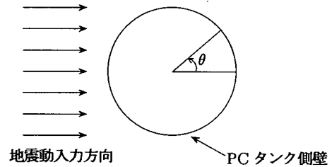
図-6 θの定義
