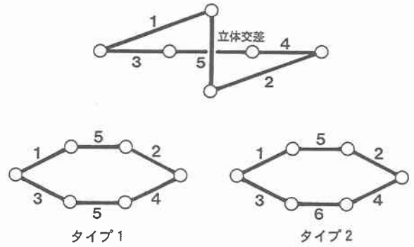
図-2 立体交差とその等価的表現
