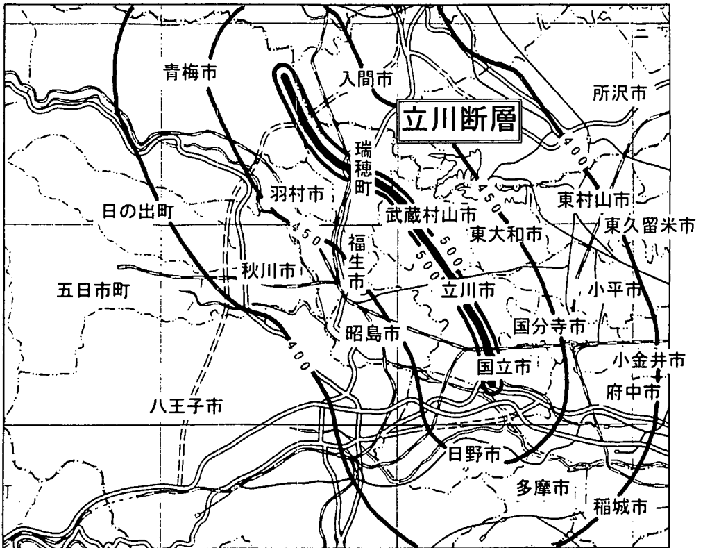
図-1 立川断層からの離れによる基盤加速度の分布図
