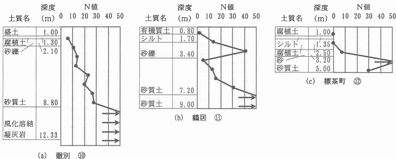
図-8(a), (b), (c) 徹別から標茶町にかけての地質柱状図 (D-D')
