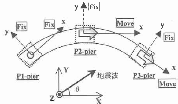
図-2 支承の配置方向と地震波の入力方向
