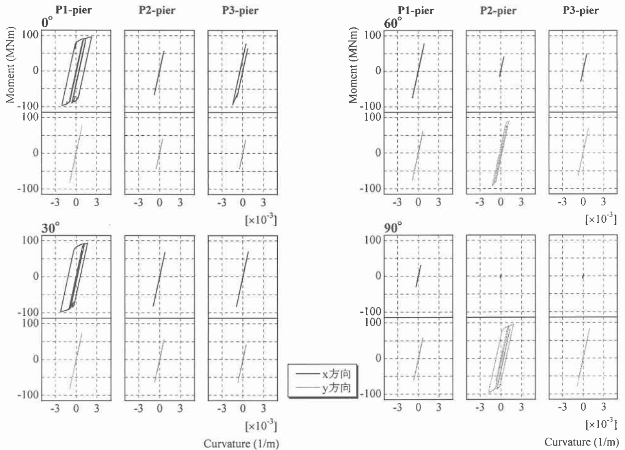
図-5 橋脚基部の曲げモーメント-曲率関係
