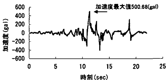
図-5 入力地震波形
