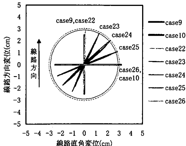
図-10 5 径間節点 1 における変位の時刻歴
