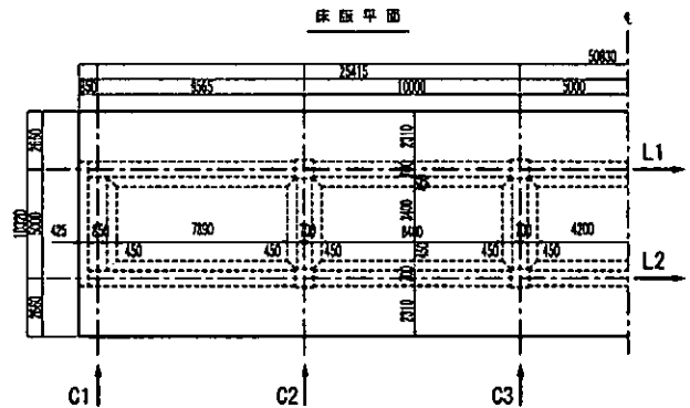
図-1 鉄道RCラーメン高架橋構造図
