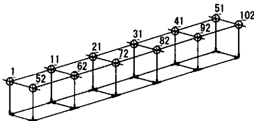
図-2 3次元解析骨組図(5径間)
