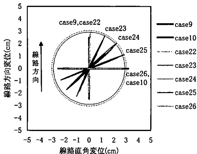
図-9 3 径間節点 1 における変位の時刻歴
