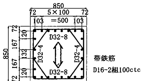
図-6 高架橋柱断面図
