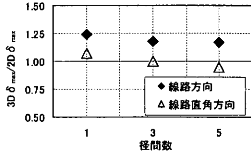
図-14 3D \delta_{max}/2D \delta_{max} と径間数の関係
