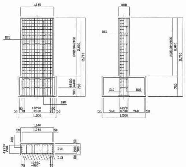
図-2 供試体形状・配筋概要図
