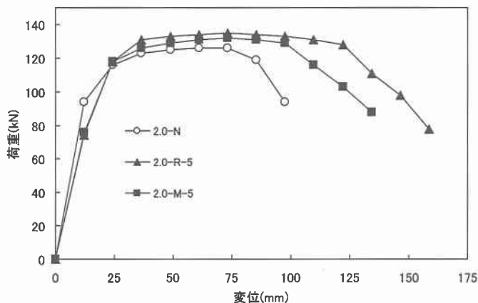
図-3 荷重-変位関係包絡線
