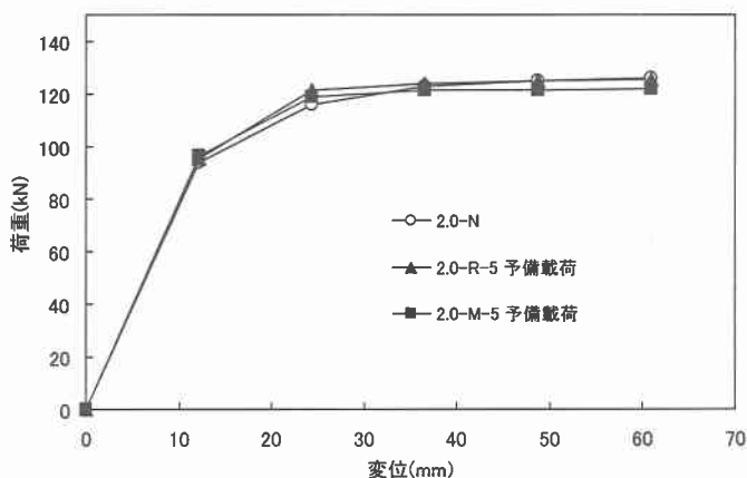
図-5 荷重-変位包絡線 (予備荷重時)
