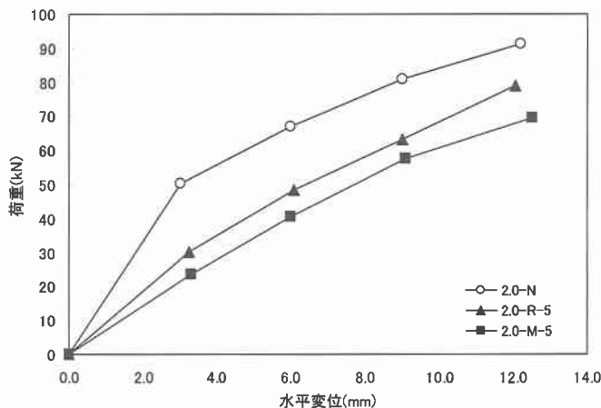
図-4 荷重-変位包絡線 (1ループ目押し Max まで)
