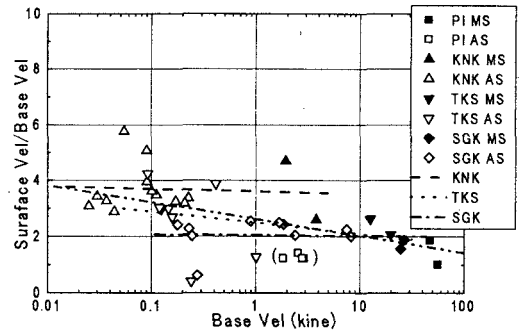
図-3 地表と基盤の間での水平速度増幅率と基盤速度の関係
