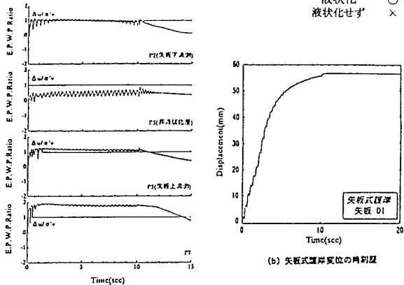
(a) 過剰間隙水圧比の時刻歴
