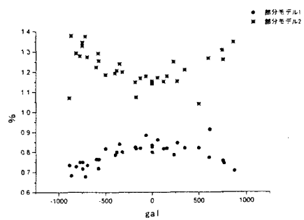
〈図4 破壊時の加速度と加速度振幅の変化率〉
