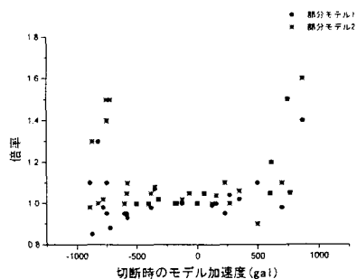
〈図7 部分モデルの速度増分〉
