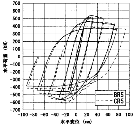
図-3 ヒステリシスループ (BR5, CR5)
