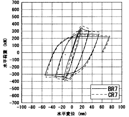
図-2 ヒステリシスループ (BR7, CR7)
