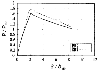
図-4 包絡線 (BR7, CR7)
