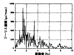
図-3 JMA 神戸波のフーリエスペクトル
