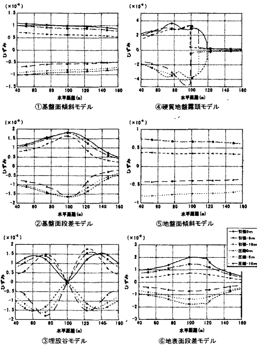
図-4 地盤ひずみ分布 (FEM)
