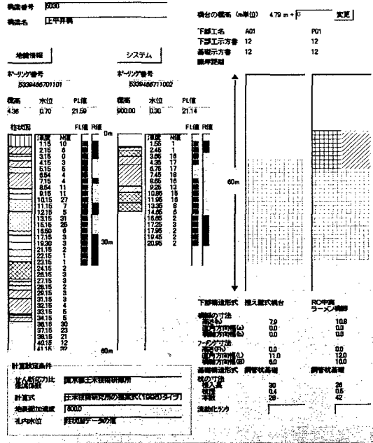
図-3 下部構造形式等一覧
