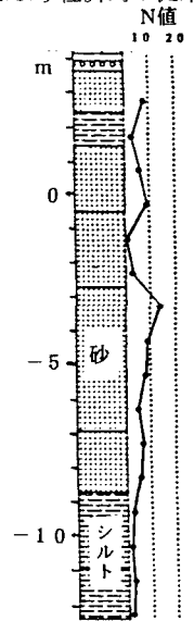
図1 土質柱状図
