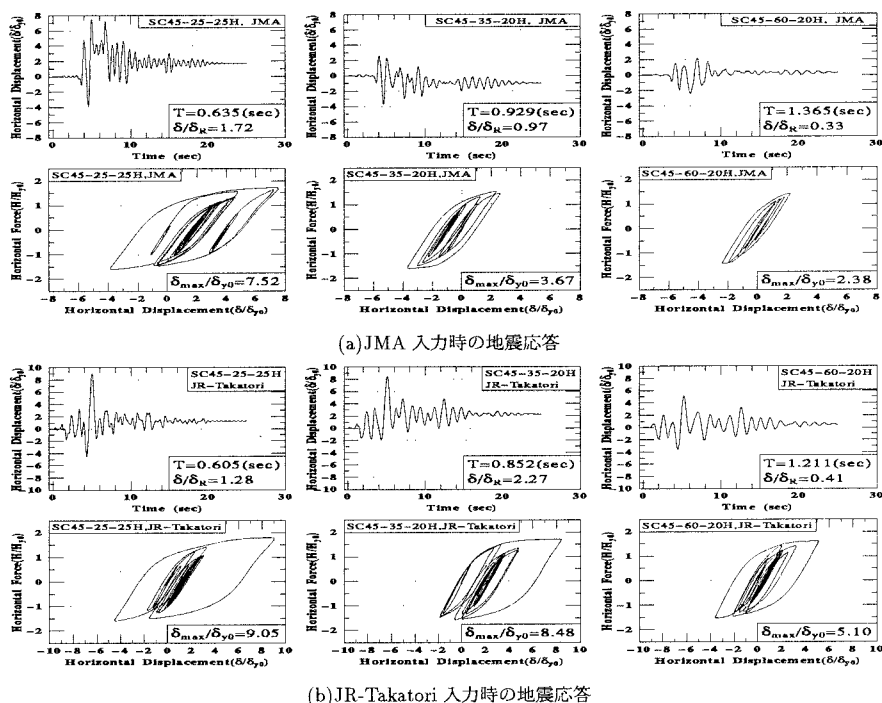
Fig. 3 コンクリート部分充填柱の時刻歴応答変位波形および復元力履歴ループ
