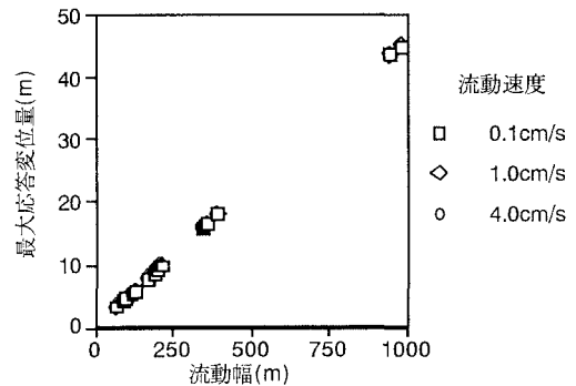
図3 地盤流動幅と管路の最大応答変位量
