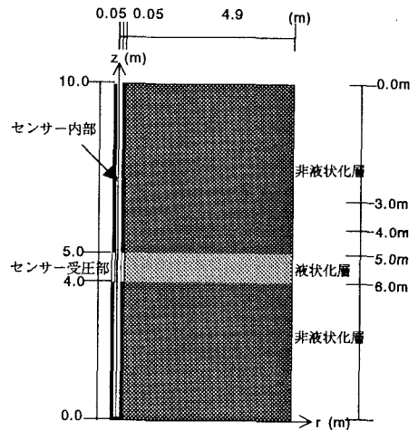
図1 軸対称地盤モデル
