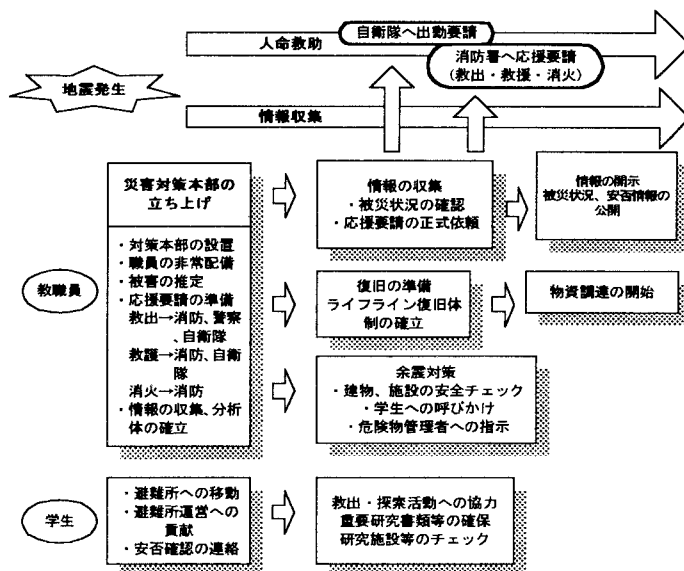
図-2 応急対策フロー概要図
