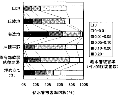
図3 代表地形による配水管・給水管被害率
