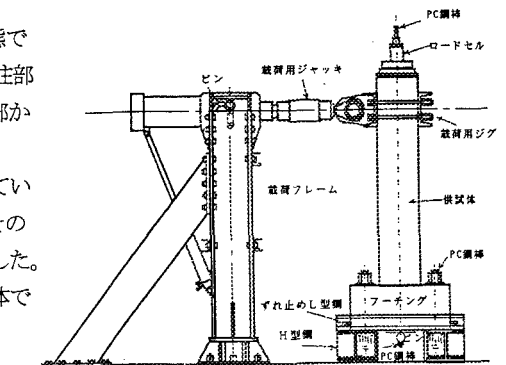
図-2 荷重装置
