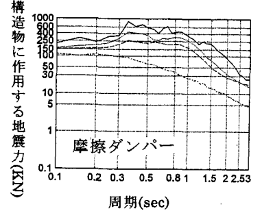
図(4.8) 構造物に働く地震力
