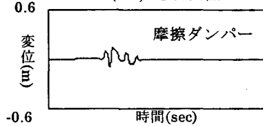
図(4.6) 応答変位
