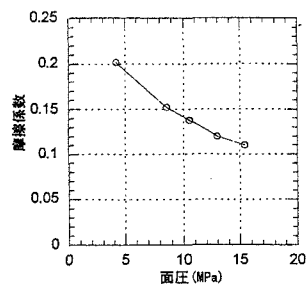
図-2. 摩擦係数の面圧依存性
