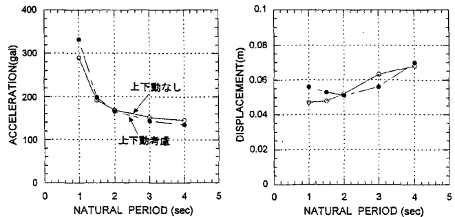
図-5. 免震効果に及ぼす上下動の影響
