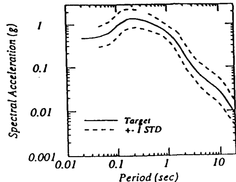
図4 平滑化された応答スペクトルの中央値とその標準偏差
