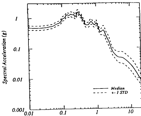
図2 全ての震源パラメータの変動を考慮した場合の応答スペクトルの中央値と標準偏差
