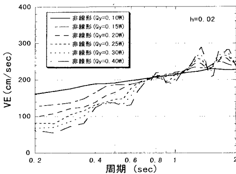
図-2 エネルギースペクトル (タイプI I種地盤 KAIHOKU BRG.LG)
