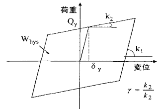
図-1 構造物の総吸収エネルギー
