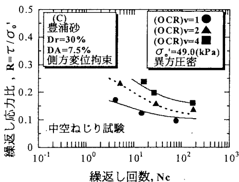
図 4 繰返し応力比と繰返し回数の関係
