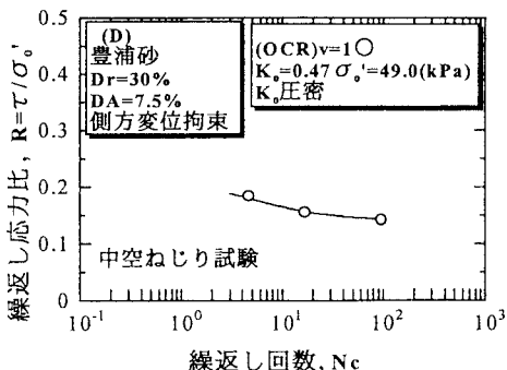
図 5 繰返し応力比と繰返し回数の関係
