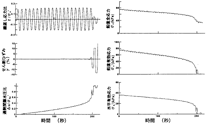
図1 ケース(B)の時刻歴
