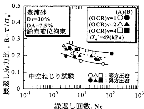
図 3 繰返し応力比と繰返し回数の関係
