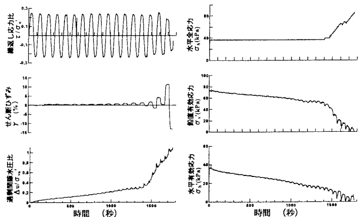
図2 ケース(C)の時刻歴
