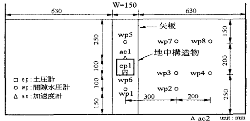
図-1 実験モデル
