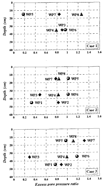
図-2 過剰間隙水圧比の最大値
