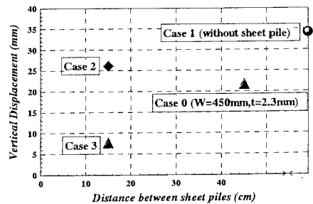
図-6 構造物浮上り量
