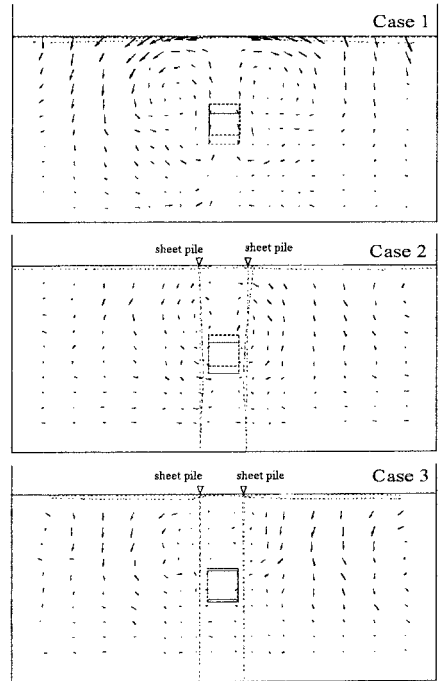
図-5 地盤変位ベクトル
