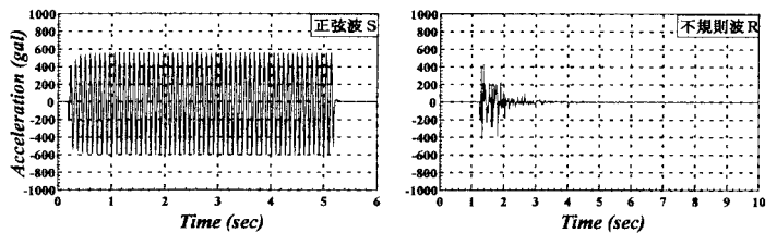
図-2 入力加速度
