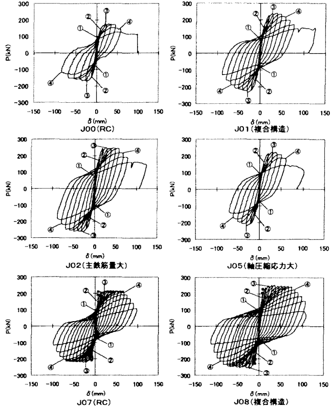
※①ひび割れ発生・②引張鉄筋降伏・③最大耐力・④かぶりコンクリート剥落
