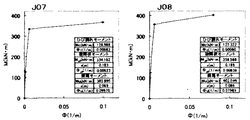
図-3 M- \Phi 骨格曲線
