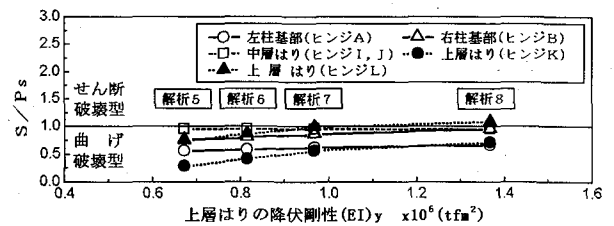
図-6 上層はりの降伏剛性と S/P_s の関係
