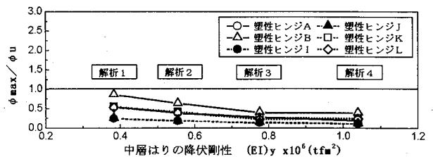
図-8 中層はりの降伏剛性と \phi_{max}/\phi_u の関係(タイプII地震動)
