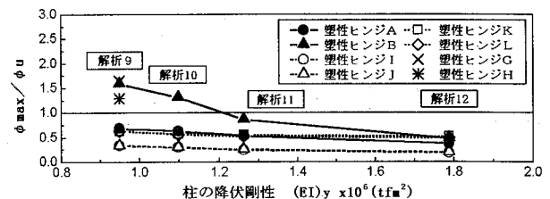
図-10 柱の降伏剛性と \phi_{max}/\phi_u の関係(タイプII地震動)
