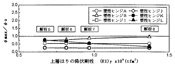
図-9 上層はりの降伏剛性と \phi_{max}/\phi_u の関係(タイプII地震動)
