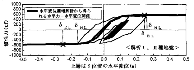
図-13 慣性力と応答変位関係
