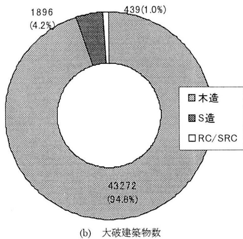
図-3.6 濃尾地震を想定した場合の損壊建築物数
