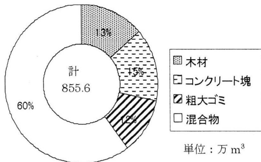
図-3.7 濃尾地震を想定した場合の解体副産物発生量
